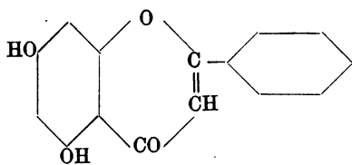
Chrysin (14).
